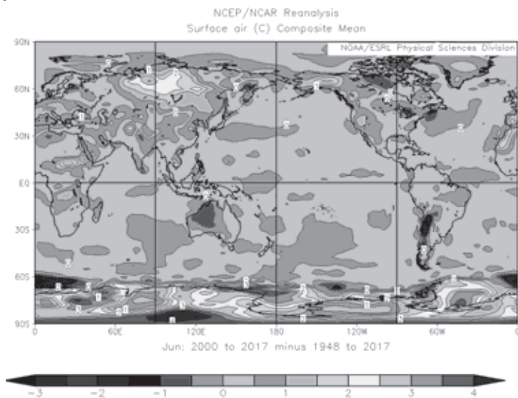
Рис.1. Карта аномалий средней месячной температуры у поверхности Земли в июне 2000–2017 гг. по сравнению с периодом 1948–2017 гг.
