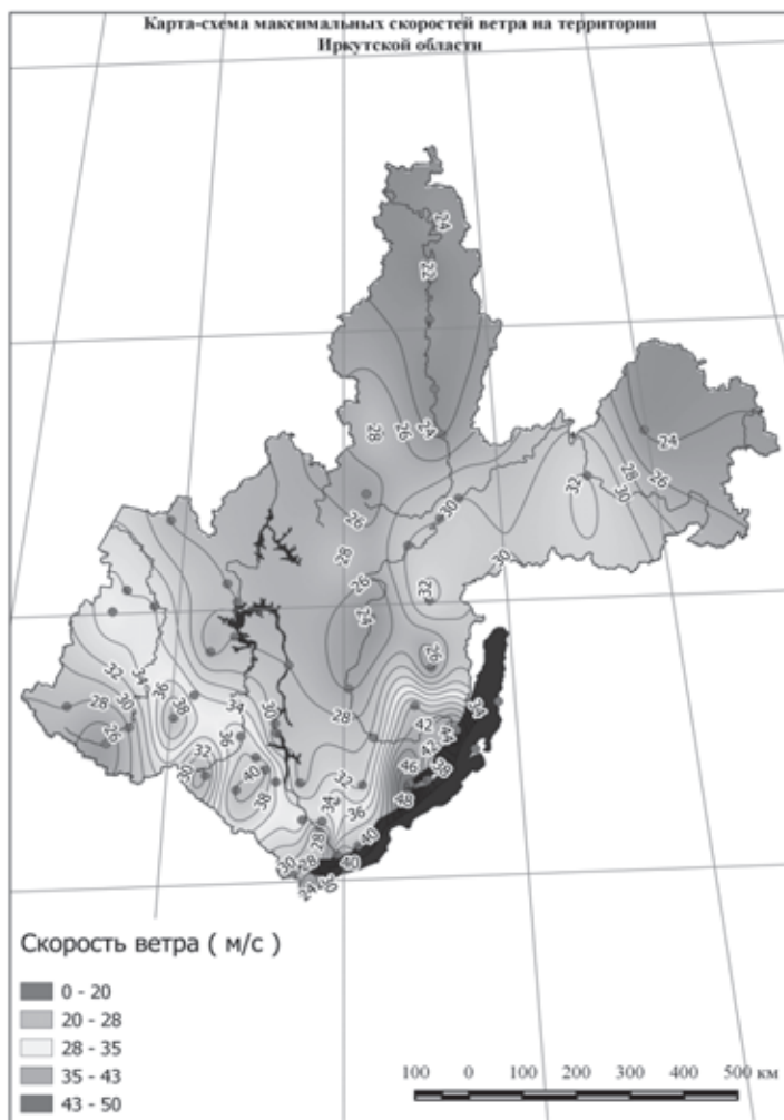
Рис.2. Карта-схема максимальной скорости ветра на территории Иркутской области за период 1961–2016 гг.
