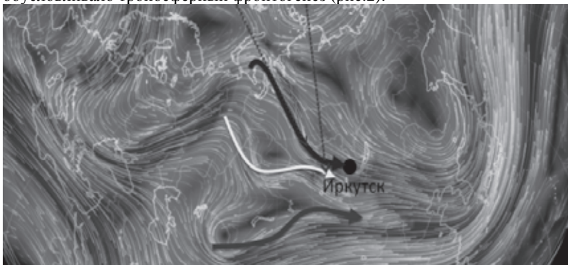
Рис.2. Карта ветровых потоков АТ–300 гПа (9 км) 19.12.2017 г. за 12 всв [2]
