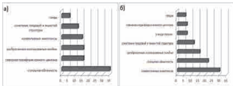
Рис.2. Повторяемость (%) различных типов мезоструктуры грозовых облаков с ливневыми осадками в г. Иркутске (а) и в горных районах Восточных Саян (б) в 2012–2017 гг.
