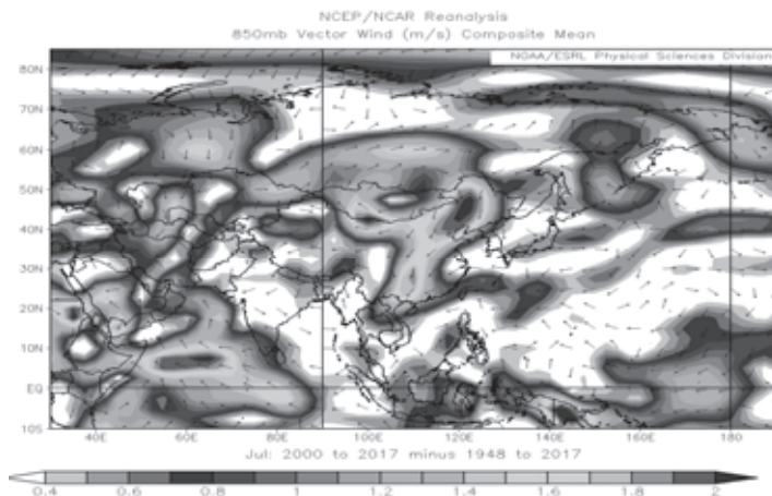
Рис.2. Карта аномалий ветровых потоков на АТ–850 гПа (1,5 км) в июле 2000–2017 гг. по сравнению с периодом 1948–2017 гг.
