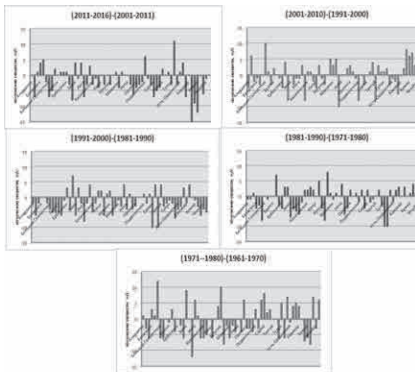
Рис.1. Изменения максимальной скорости ветра (м/с) на метеорологических станциях Иркутской области между различными временными периодами
