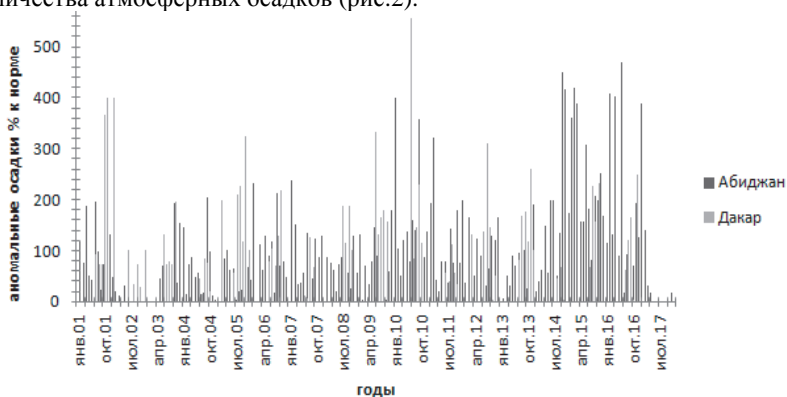
Рис.2. Аномалии месячных сумм атмосферных осадков (% к норме) на ст. Абиджан и Дакар в 2001–2017 гг.
