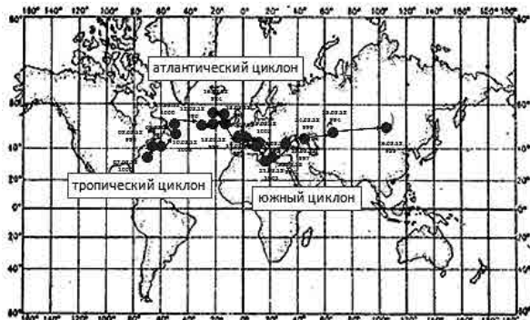
Рис.1. Траектория смещения циклона, который образовался 07.03.2018 г. и 26.03.2018 г. сместился на территорию Иркутской области
