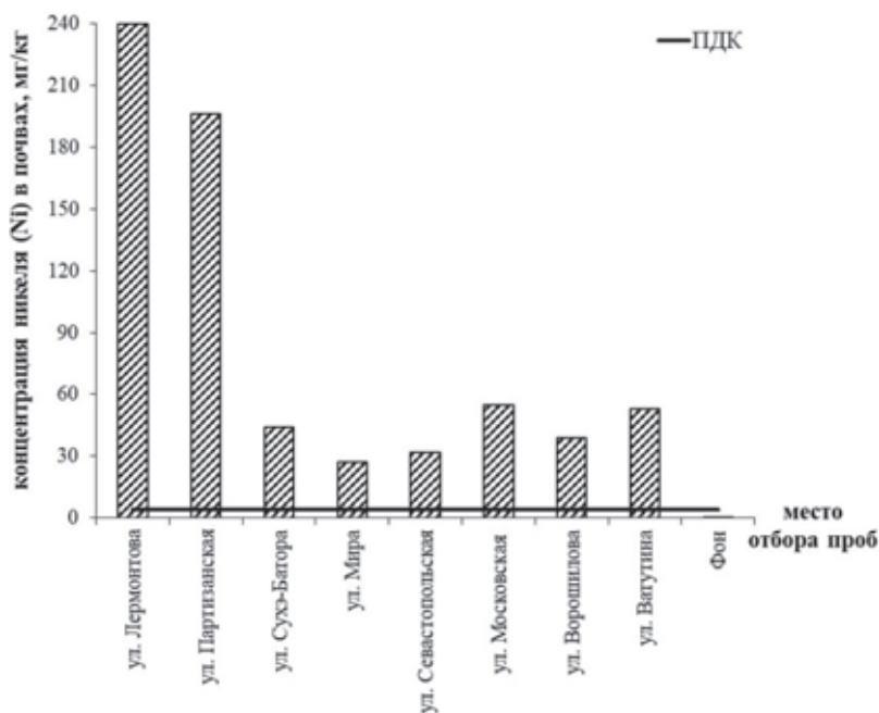
Рис. 1. Концентрация никеля в отобранных образцах почв
