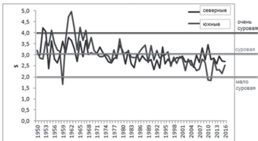
Рис.2. Изменение средних значений индекса суровости зим в северных и южных районах Иркутской области в январе 1950–2016 гг.
