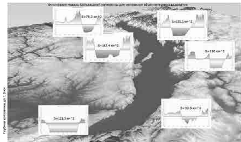
Рис. 2. Физическая модель Байкальской котловины
