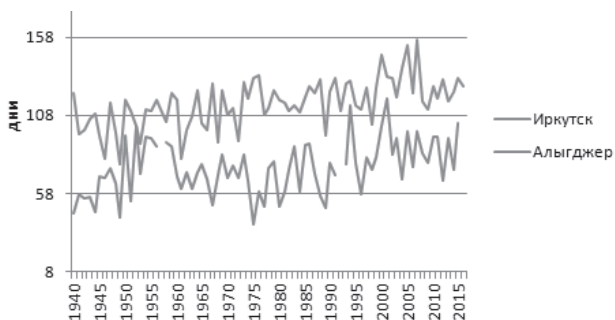
Рис.2. Изменение продолжительности безморозного периода (дни) на станциях Иркутск и Алыгджер в 1940–2016 гг.
